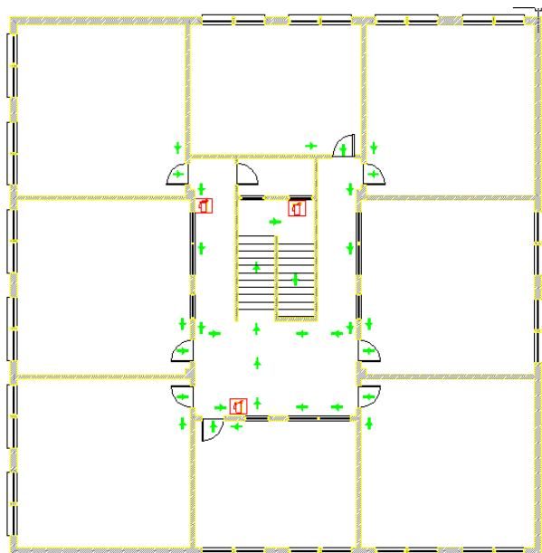
Parte da Planta de Evacuação do 1º Andar do Bloco B
